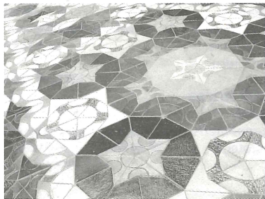
Mosaico de Penrose. Sala de Matemáticas
